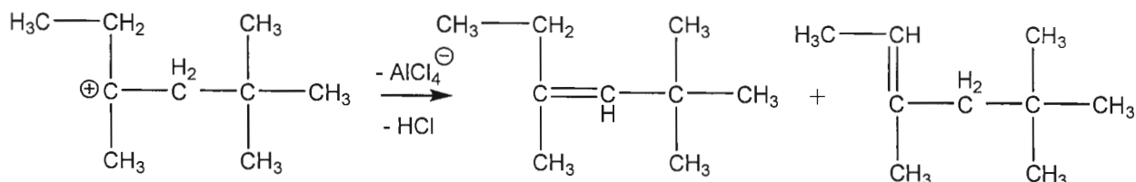
Г - 2,2,4-триметилгексен-3 или 3,5,5-триметилгексен-2
