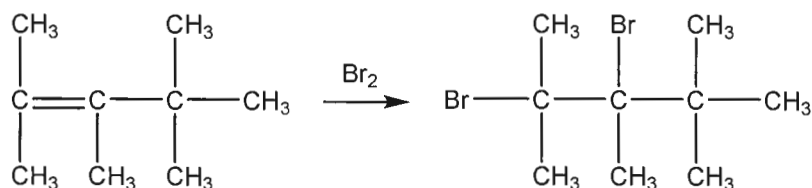
Ж - 2,3-дибром-2,3,4,4-тетраметилпентан
