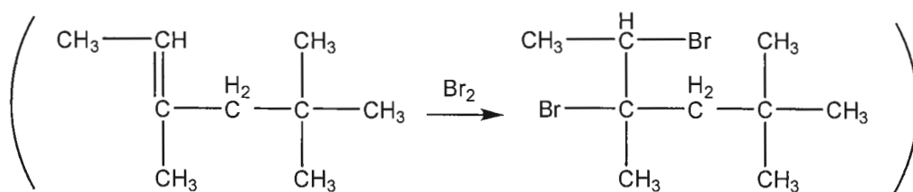
Или Е - 2,3-дибром-3,5,5-триметилгексан
