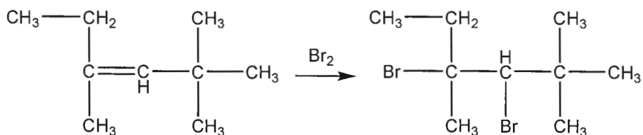
Е - 3,4-дибром-2,2,4-триметилгексан
